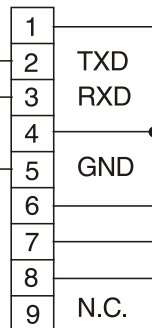
Abbildung 4-5. Verbindungen vom PC zum DECS-100
