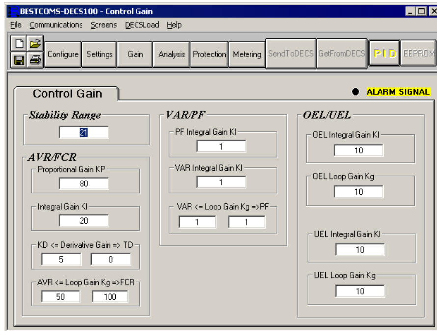
Abbildung 5-9. Fenster Steuerverstärkung
