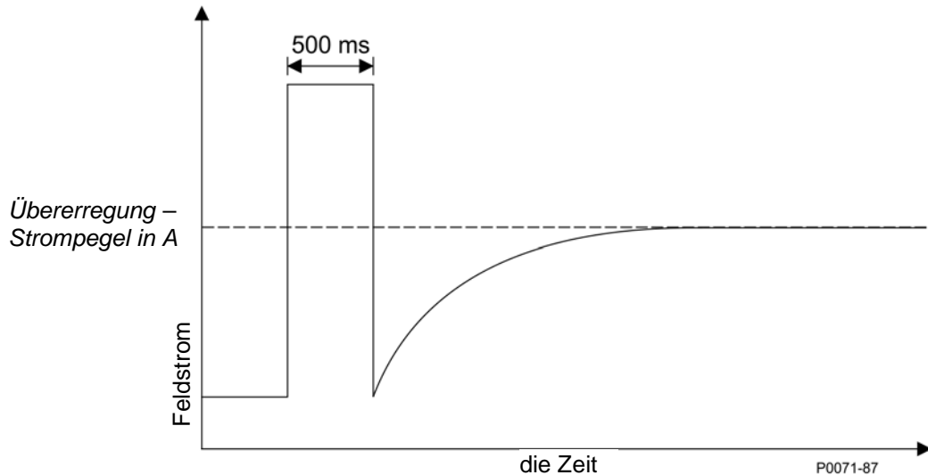
Abbildung 3-2. Zeitkennlinie, Übernahme-OEL
