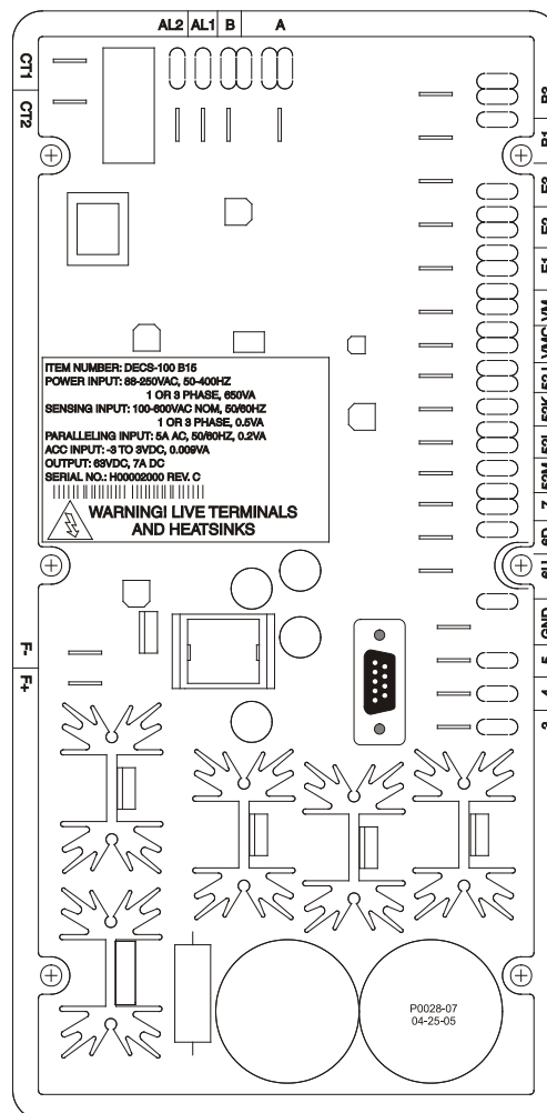
Abbildung 4-3. DECS-100 Anschlussklemmen
