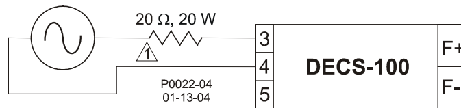
Abbildung 4-12. Betriebsleistungsanschlüsse für die DECS-100-Programmierung (Eingangsspannung >120 Vac)
