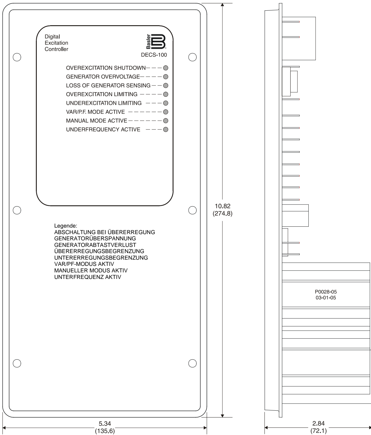
Abbildung 4-1. DECS-100 Abmessungen
