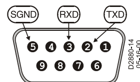
Figure 4-4. Affectations des broches du port RS-232
