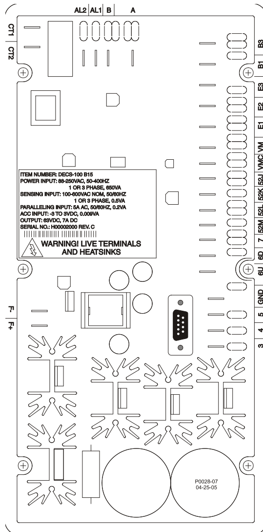
图 4-3. DECS-100 端子
