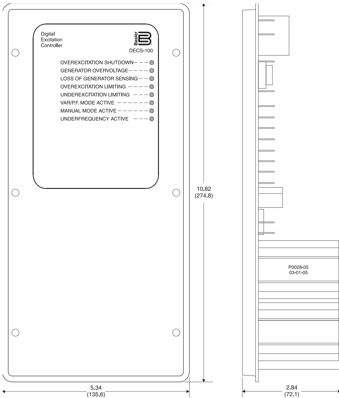
图 4-1. DECS-100 尺寸
