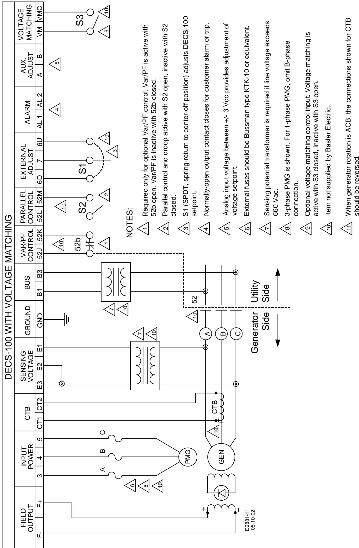
图 4-7. PMG,ABC 相序, 单相检测典型接线图
