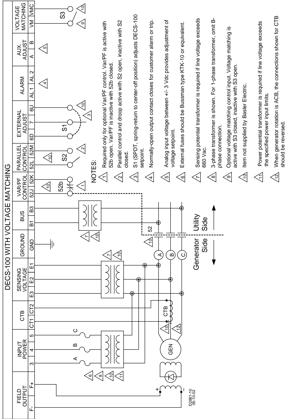
图 4-8. 励磁, ABC 相序, 三相检测典型接线图
